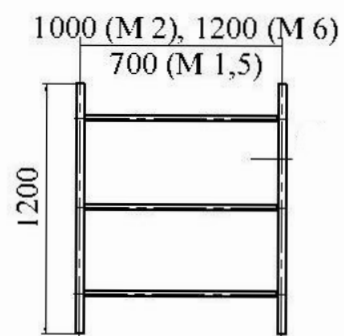
рама рядовая М 1,2,5,6 (3) синяя рама ограждения М 1,2,5,6 (6) красная
